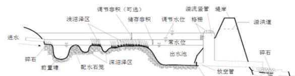
雨水湿地典型构造图
