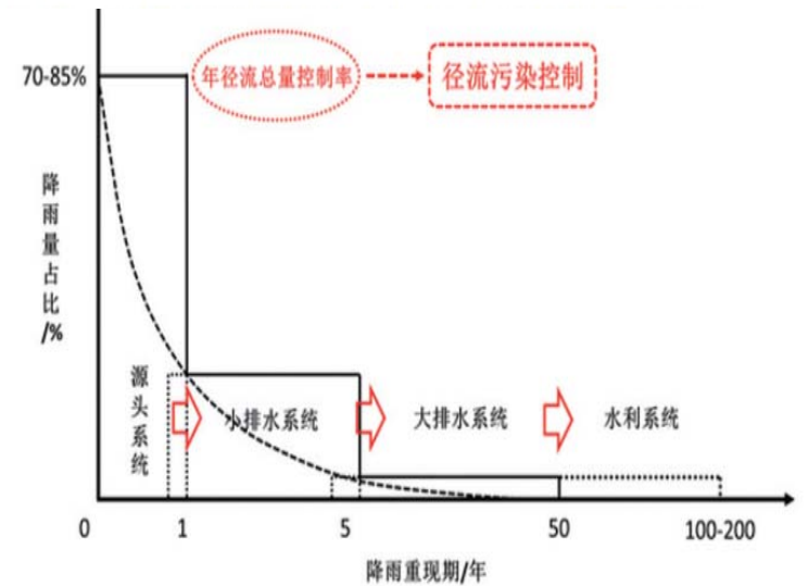
大-小-微+城市水利系统中 径流总量、径流污染控制示意图
